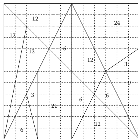
Figura 2. Puzzle Stomachion sobre cuadrícula
